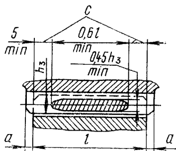
Рис. 195. Пятно контакта ведомой цилиндрической шестерни: a — разность указанных размеров \max 10
