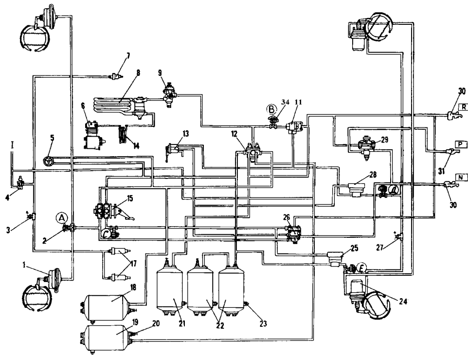
Рис. 289. Схема пневматического привода тормозных механизмов автомобилей КамАЗ-4326: 1 - тормозные камеры типа 24; 2 (А, В, С) - контрольные выходы; 3 - пневмоэлектрический выключатель электромагнитного клапана прицепа; 4 - кран управления вспомогательной тормозной системой; 5 - двухстрелочный манометр; 6 - компрессор; 7 - пневмоцилиндр привода рычага останова двигателя; 8 - водоотделитель; 9 - регулятор давления; 11 - двухмагистральный перепускной клапан; 12 - 4-х контурный защитный клапан; 13 - кран управления стояночной тормозной системой; 14 - теплообменник; 15 - двухсекционный тормозной кран; 17 - пневмоцилиндры привода заслонок механизма вспомогательной тормозной системы; 18 - ресивер контура I; 19 - ресивер потребителей; 20 - выключатель сигнализатора падения давления; 21 - ресивер контура III; 22 - ресиверы контура II; 23 - кран слива конденсата; 24 - тормозные камеры типа 20/20 с пружинными энергоаккумуляторами; 25, 28 - ускорительные клапаны; 26 - клапан управления тормозными системами прицепа с двухпроводным приводом; 27 - выключатель сигнализатора стояночной тормозной системы; 29 - клапан управления тормозными системами прицепа с однопроводным приводом; 30 - автоматические соединительные головки; 31 - соединительная головка типа А; R - к питающей магистрали двухпроводного привода; P - к соединительной магистрали однопроводного привода; N - к управляющей магистрали двухпроводного привода; 31 - датчик падения давления в ресиверах I контура; 32 - датчик падения давления в ресиверах II контура; 33 - датчик стоп- сигнала; 34 - кран экстренного растормаживания
