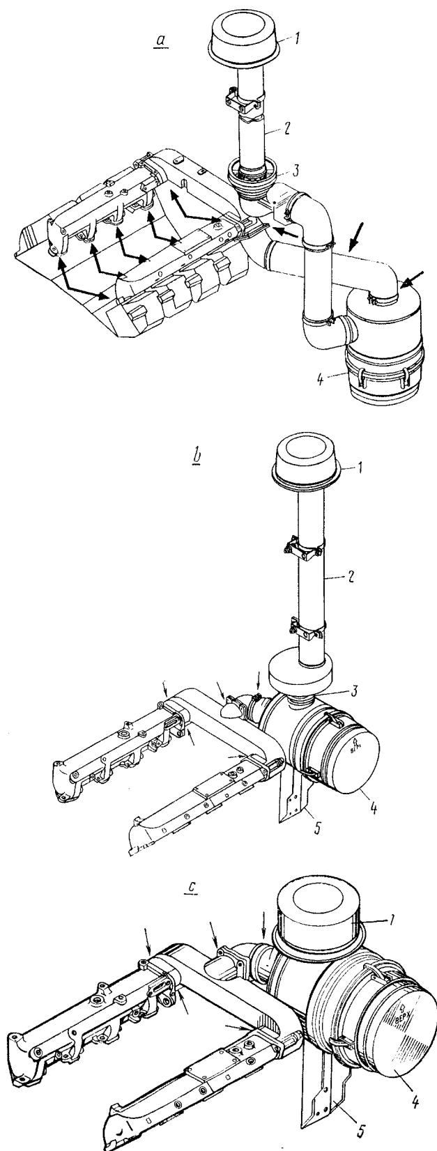
Рис. 47. Схема систем забора воздуха автомобилей: а - моделей 5320 и 55102; б - моделей 53212, 5410 и 54112; в - модели 55111; 1 - колпак; 2 - труба воздухозаборника; 3 - уплотнитель; 4 - воздухоочиститель; 5 - кронштейн (стрелками указаны места, подлежащие контролю герметичности при обслуживании системы)
