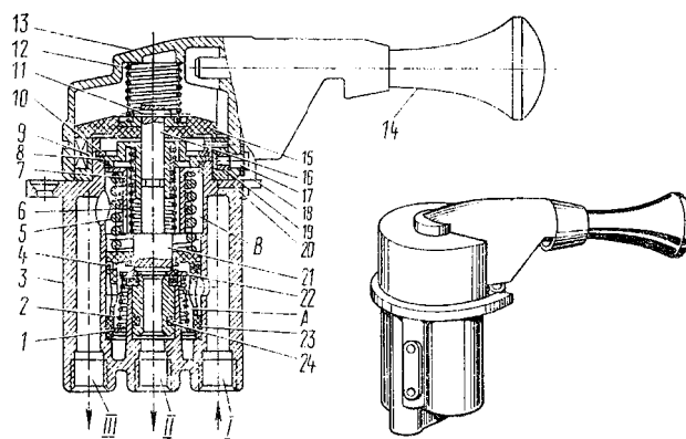
Рис. 301. Кран управления стояночной тормозной системой: 1, 10 - кольца упорные; 2 - пружина клапана; 3 - корпус; 4, 24 - кольца уплотнительные; 5 - пружина уравнивающая; 6 - пружина штока; 7 - тарелка уравнивающая; 8 - направляющая штока; 9 - кольцо фигурное; 11 - штифт; 12 - пружина колпачка; 13 - крышка; 14 - рукоятка крана; 15 - колпачок направляющий; 16 - шток; 17 - ось ролика; 18 - фиксатор; 19 - ролик; 20 - стопор; 21 - седло выпускное клапана на штоке; 22 - клапан; 23 - поршень следящий; I - от ресивера; II - в атмосферу; III - в управляющую магистраль ускорительного клапана
