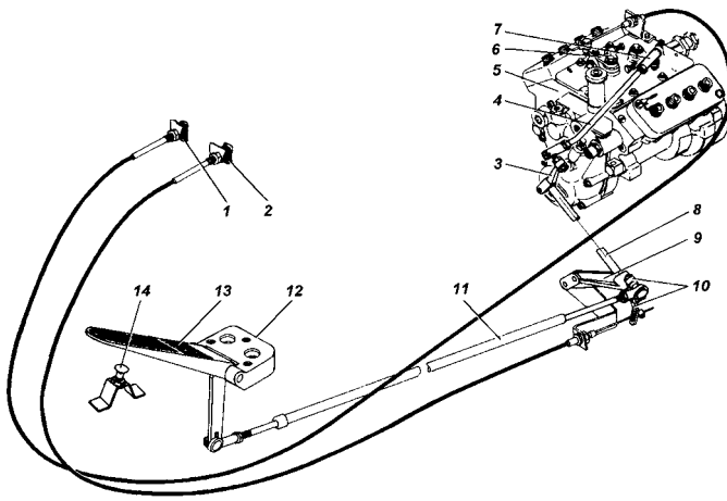
Рис. 45. Привод управления подачей топлива: 1-рукоятка тяги останова двигателя; 2-рукоятка тяги ручного управления подачей топлива; 3, 10-задние рычаги; 4-тяги рычага управления регулятором; 5-ТНВД; 6-рычаг останова двигателя; 7-рычаг управления регулятором; 8-поперечный валик; 9-задний кронштейн; 11-телескопическая тяга; 12-кронштейн педали; 13-педаль; 14-регулирующий болт
