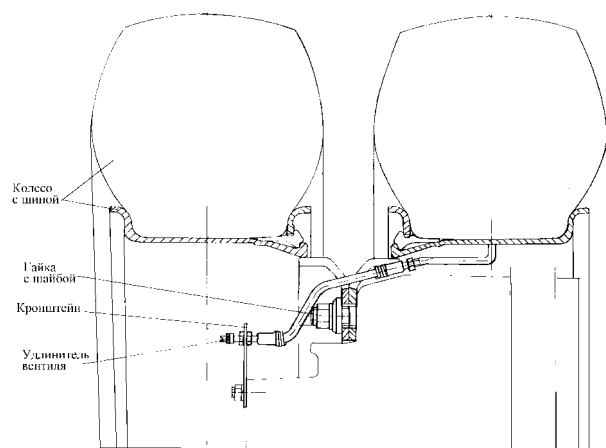
Рис. 217. Колеса дисковые сдвоенные
