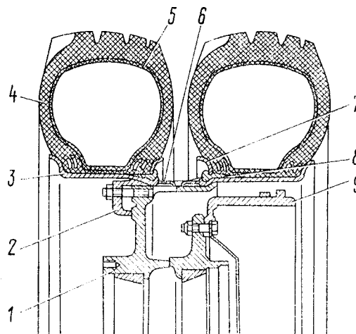
Рис. 214. Колесо с балансировочными грузами: 1 - обод колеса; 2 - кольцо замочное; 3 - кольцо бортовое; 4 - груз балансировочный в сборе; 5 - шина; 6 - камера; 7 - лента ободная; 8 - заклепка; 9 - груз балансировочный; 10 - пружина
