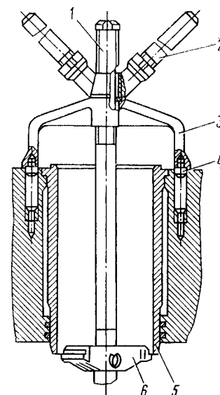
Рис. 81. Снятие гильзы цилиндра съемником И801.05.000: 1 - винт; 2 - рукоятка; 3 - корпус; 4 - опора; 5 - гильза; 6 - захват
