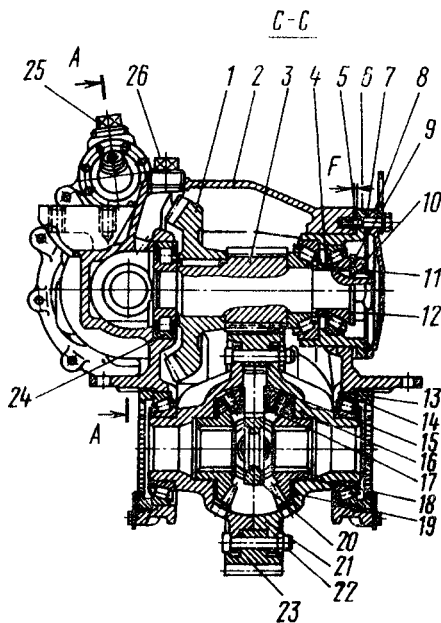
Рис. 190. Главная передача промежуточного моста: 1 - шестерня ведомая коническая; 2 - картер главной передачи; 3 - шестерня ведущая цилиндрическая; 4, 44 - шайбы регулировочные; 5, 29 - прокладки регулировочные; 6 - стакан; 7, 33 - прокладки; 8 - крышка; 9, 15, 19 - шайбы опорные; 10 - гайка подшипника; 11, 12, 14, 42, 45 - подшипники роликовые конические; 13 - гайка регулировочная; 16 - сателлит; 17 - втулка сателлита; 18 - шестерня полуосевая; 20 - крестовина; 21 - чашка дифференциала; 22 - болт крепления чашек дифференциала; 23 - шестерня ведомая цилиндрическая; 24 - подшипник роликовый цилиндрический; 25, 26 - пробки заливные; 27 - картер межосевого дифференциала; 28 - стакан; 30 - шестерня ведущая коническая; 31 - вал задний; 32 - подшипник шариковый; 34 - крышка; 35 - манжета; 36 - отражатель; 37 - фланец; 38 - гайка; 39 - шайба; 40 - крышка подшипника дифференциала; 41 - стопор; 43 - втулка распорная
