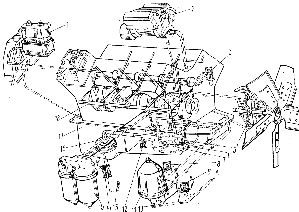
Рис. 30. Схема системы смазывания: 1 - компрессор; 2 - насос топливный высокого давления; 3 - выключатель гидромфты; 4 - гидромфта; 5, 12 - клапаны предохранительные; 6 - клапан системы смазывания; 7 - насос масляный; 8 - клапан перепускной центробежного фильтра; 9 - клапан сливной центробежного фильтра; 10 - кран включения масляного радиатора; 11 - фильтр центробежный; 13 - лампа сигнальная засоренности фильтра очистки масла; 14 - клапан перепускной фильтра очистки масла; 15 - фильтр очистки масла; 16 - маслоприемник; 17 - картер; 18 - магистраль главная; А - в радиатор
