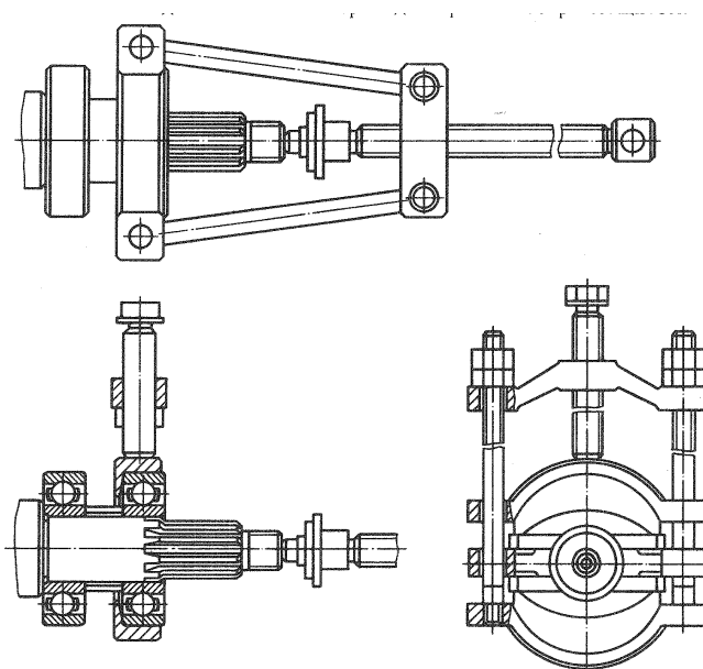
Рис. 168. Снятие подшипников вала привода коробки отбора мощности
