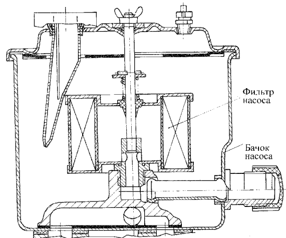
Рис. 279. Фильтр насоса гидроусилителя руля
