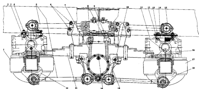
Рис. 205. Установка задней подвески (продольный вид) 43101, 43114, 43118: 1 - мост промежуточный; 2 - рама; 3 - рычаг реактивный верхний; 4 - шпильки; 5 - штанги реактивные; 6, 10, 13 - болты; 7 - стремянка рессоры; 8 - накладка рессоры; 9 - гайка стремянки; 11 - палец опоры; 12 - подкладка буфера; 14 - буфер; 15 - крышка шарового пальца; 16 - опора; 17 - мост задний; 18, 22 - рычаги реактивные нижние; 19 - кронштейн оси балансира; 20 - пробка заливного отверстия; 21 - рессора
