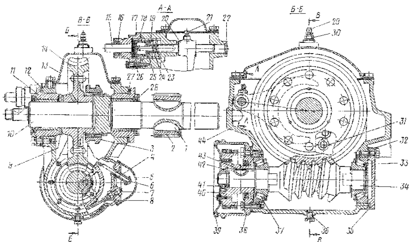
Рис. 237. Редуктор лебедки: 1—шлицевая втулка; 2, 43—шпонки; 3—муфта включения; 4, 23, 24—пружины; 5—крышка пружины; 6, 7, 41—гайки; 8—лента тормозного механизма; 9, 42—упорные шайбы; 10—вал барабана; 11— стакан; 12, 18, 27, 35—прокладки; 13— крышка картера; 14—червячное колесо; 15—упорный палец штока; 16—сальник; 17— крышка штока; 19—шток вилки; 20—вилка включения; 21— уст ановочный винт; 22— заглушка; 25— стакан штока; 26— крышка; 28— манжета; 29— предохранительный клапан; 30— переходник; 31— болт; 32— крышка заднего подшипника; 33, 37—подшипники; 34—червяк редуктора; 36—пробка; 38— крышка переднего подшипника; 39— отражатель барабана; 40—барабан тормозного механизма; 44—картер редуктора лебедки
