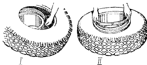
Рис. 234. Монтаж шины
