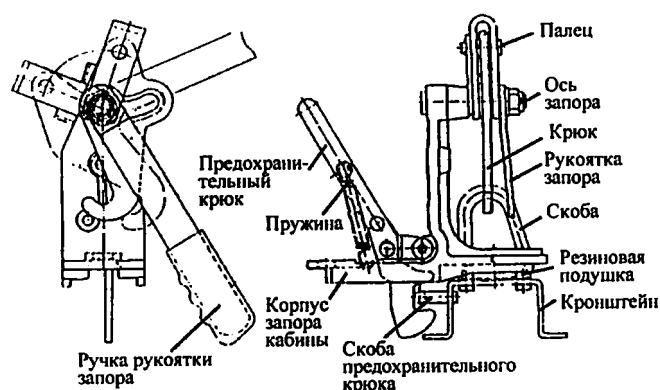
Рис. 247. Запорное устройство кабины
