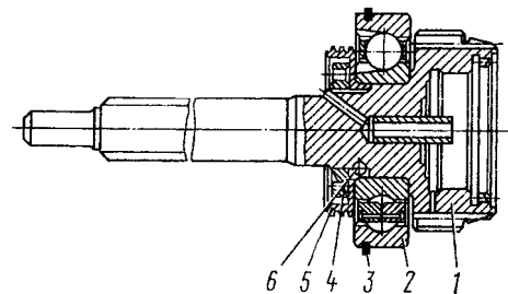
Рис. 130. Ведущий вал в сборе: 1 - вал ведущий; 2 - подшипник шариковый; 3 - кольцо стопорное подшипника; 4 - гайка кольцевая; 5 - кольцо маслоснабжающее; 6 - шарик стопорный
