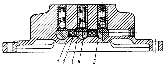
Рис. 134. Замок и фиксаторы механизма переключения: 1 - шарик замка; 2 - стакан стопорного шарика; 3 - пружина стопорного шарика; 4 - штифт замка; 5 - шарик стопорный фиксатора
