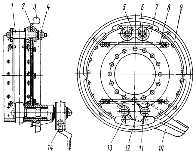
Рис. 285. Тормозной механизм: 1 - ось колодки; 2 - суппорт; 3 - щиток; 4 - гайка оси; 5 - накладка осей колодок; 6 - чека оси колодки; 7 - колодка тормозная; 8 - пружина; 9 - накладка фрикционная; 10 - кронштейн разжимного кулака; 11 - ось ролика; 12 - кулак разжимной; 13 - ролик; 14 - рычаг регулировочный
