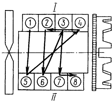
Рис. 19. Схема нумерации и порядок работы цилиндров: 1...8 - цилиндры; I - правый ряд; II - левый ряд
