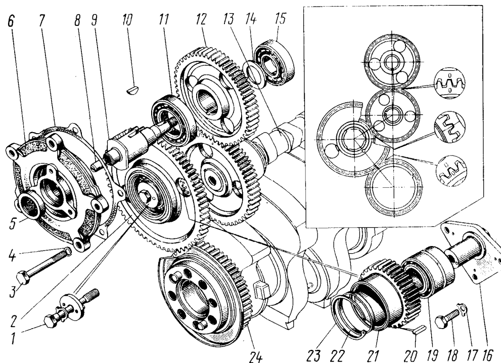
Рис. 22. Шестерня привода генератора: 1 - болт M12x1,25x90 крепления роликового подшипника; 2, 21 - шестерни промежуточные; 3-болт; 4 - шайба пружинная; 5-манжета; 6-корпус заднего подшипника; 7-прокладка; 8 - сухарь; 9 - вал шестерни привода топливного насоса высокого давления; 10, 20 - шпонки; 11, 15 - подшипники шариковые; 12 - шестерня привода топливного насоса высокого давления; 13-вал распределительный в сборе с шестерней; 14 - шайба упорная; 16 - ось ведущей шестерни; 17 - шайба; 18 - болт M10x1,25x25; 19 - подшипник роликовый конический двухрядный; 22 - кольцо упорное; 23 - кольцо стопорное; 24 - шестерня ведущая коленчатого вала
