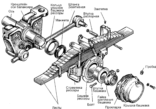
Рис. 208. Подвеска задняя
