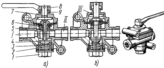
Рис. 317. Разобистельный кран: а - кран открыт; б - кран закрыт; 1 - пробка; 2 - корпус; 3 - пружина клапана; 4 - клапан; 5 - пружина штока; 6 - шток с мембраной; 7 - крышка; 8 - толкатель; 9 - рукоятка; I - к соединительной головке; II - от ресивера; III - в атмосферу
