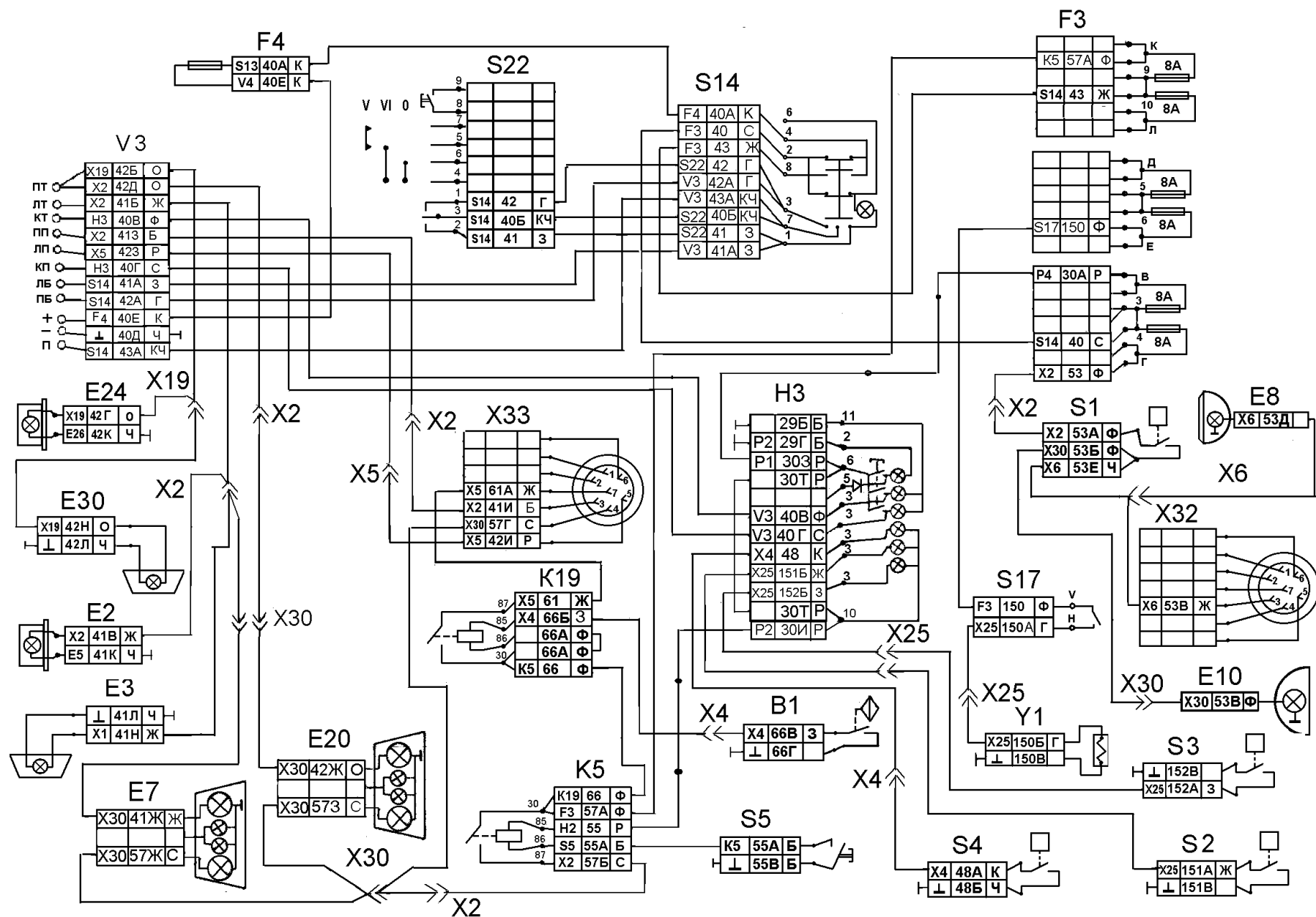
Рис. 335. Функциональная схема наружной световой сигнализации и блокировки колес. Распространяется на все автомобили
