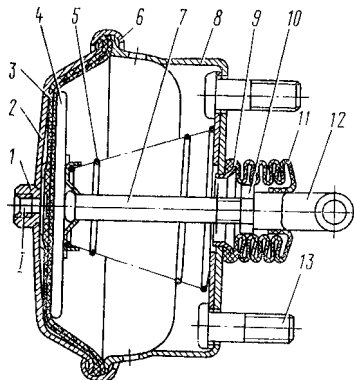
Рис. 309. Тормозная камера типа 24: 1 - штуцер; 2 - крышка корпуса; 3 - мембрана; 4 - диск опорный; 5 - пружина возвратная; 6 - хомут; 7 - шток; 8 - корпус камеры; 9 - кольцо; 10 - контргайка; 11 - чехол защитный; 12 - вилка; 13 - болт; 1 - подвод сжатого воздуха
