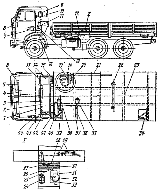
Рис. 359. Схема размещения инструмента и принадлежностей: 1 - ящик для запасных частей; 2 - индивидуальные средства защиты* водителя; 8 - футляр медицинской аптечки; 4 - держатель ПНВ**; 5 - держатель ДП-ЗБ**; 6 - противосолнечные козырьки; 7 - огнетушитель**; 8 - утеплитель передней части; 9 - ящик для запасных частей (автомобиль мод. 53212 со спальным местом); 10 - футляр медицинской аптечки (автомобиль мод. 53212 со спальным местом); 11 - знак аварийной остановки; 12 - инструментальный ящик; 18 - держатель ФВУ** (автомобиль мод. 5320); 14 - держатель ФВУ (автомобиль мод. 53212); 15 - КС-20 (автомобиль мод. 5320); 16 - подпятник**; 17 - запасное колесо; 18 - держатель СМУ; 19 - бачок для питьевой воды**; 20 - держатель противоткатного клина**; 21 - санитарные носилки*; 22 - держатель жесткого буксира**; 23 - установка фонаря подкузовной подсветки; 24 - гидравлический домкрат; 25 - переносная лампа; 26 - шинный манометр; 27 - топливоподкачивающий насос; 28 - шланг для прокачивания гидросистемы; 29 - смазочный шприц; 30 - шланг для накачивания шин; 31 - комплект инструмента с малой сумкой; 32 - брезентовое ведро**; 33 - комплект инструмента с большой сумкой; 34 - КС-20** (автомобиль мод. 5320); 35 - пила** (автомобиль мод. 5320); 36 - лопата**; 37 - топор**; 38 - пила** (автомобиль мод. 53212); 39 - КС-10** (автомобиль мод. 5320); 40 - держатель ДК-4Д**; 41 - КС-10** (автомобиль мод. 53212); 42 - держатель ПНВ** (автомобиль мод. 53212 со спальным местом); 43 - запасной зажим; 44 - цепи противоскольжения**
