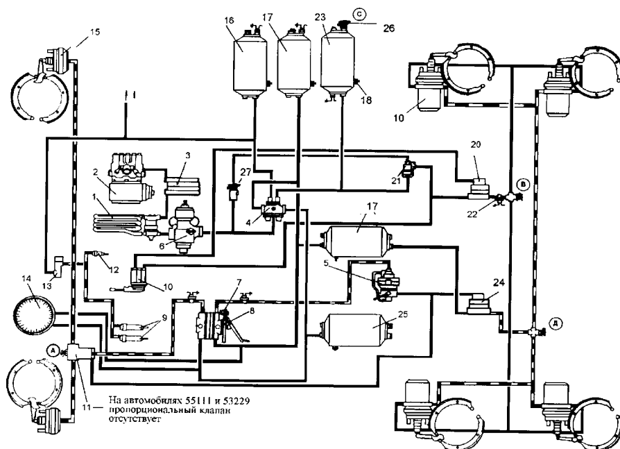
Рис. 288. Схема пневматического привода тормозных механизмов автомобилей КамАЗ-53229, -65115, -54115, -43253.1: 1 - водоотделитель; 2 - компрессор; 3 - охладитель; 4 - четырехконтурный защитный клапан; 5 - автоматический регулятор тормозных сил; 6 - регулятор давления; 7 - выключатель сигнала торможения; 8 - тормозной кран; 9 - пневмоцилиндры привода заслонки механизма вспомогательной тормозной системы; 10 - кран управления стояночной тормозной системой; 11 - пропорциональный клапан; 12 - пневмоцилиндр привода рычага останова двигателя; 13 - кран управления вспомогательной тормозной системой; 14 - манометр; 15 - тормозные камеры типа 30/30; 16 - ресивер контура IY; 17 - ресиверы контура II; 18 - кран слива конденсата; 19 - тормозные камеры типа 20/20; 20, 24 - ускорительные клапаны; 21 - двухмагистральный перепускной клапан; 26 - выключатель контрольной лампы стояночной тормозной системы; 23 - ресивер контура III; 25 - ресивер контура I; 26 - выключатель контрольной лампы падения давления воздуха в контуре III; 27 - кран экстренного растормаживания
