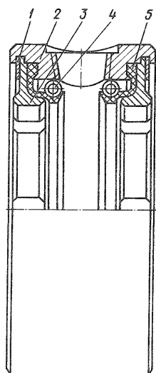
Рис. 227. Головка подвода воздуха: 1 — пружинное кольцо; 2 — корпус головки; 3 — крышка головки; 4 — пружина манжеты; 5 — набивка манжеты
