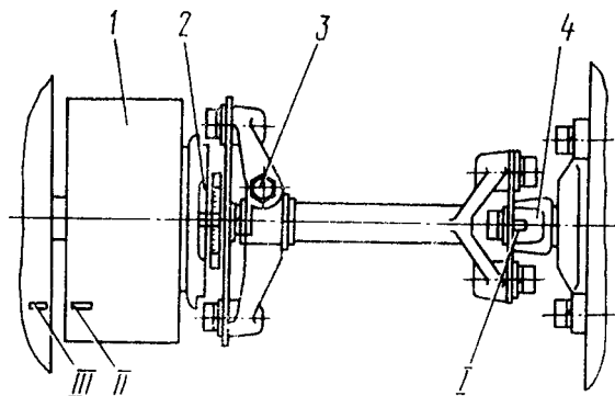
Рис. 65. Установка начала впрыскивания топлива в первом цилиндре двигателя по меткам: I - муфта автоматическая опережения впрыскивания; 2 - полумуфта ведомая; 3 - болт стяжной; 4 - фланец задний ведущей полумуфты; I - метка на заднем фланце полумуфты; II - метка на муфте опережения впрыскивания; III - метка на корпусе топливного насоса высокого давления
