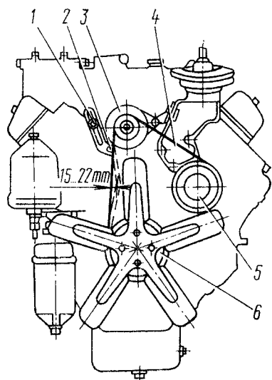
Рис. 75. Схема проверки натяжения ремней привода генератора и водяного насоса: 1 - болт; 2 - болт крепления планки; 3 - генератор; 4 - ремни привода; 5 - шкив водяного насоса; 6 - шкив гидромфты
