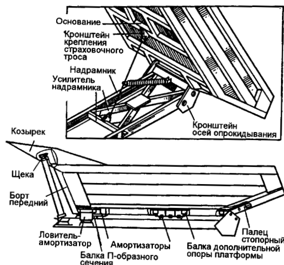
Рис. 262. Платформа автомобиля-самосвала
