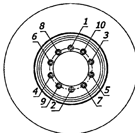
Рис. 220. Порядок затяжки гаек колеса
