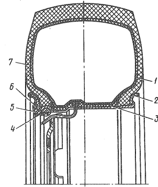
Рис. 224. Колесо с шиной в сборе: 1 — камера; 2 — бортовое кольцо; 3 — ободная лента; 4 — балансировочный груз; 5 — обод колеса; 6 — замочное кольцо; 7 — покрывка
