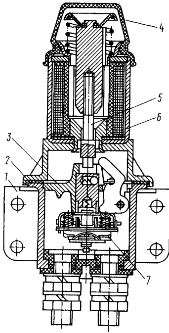
Рис. 354. Выключатель тока типа ВК-860-В: 1 - корпус; 2 - прокладка уплотнительная; 3 - плита опорная; 4 - устройство ручного включения с защитным чехлом; 5 - шток; 6 - электромагнит; 7 - система контактная
