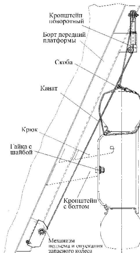
Рис. 219. Установка запасного колеса самосвала
