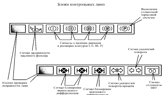
Рис. 6. Блок контрольных ламп
