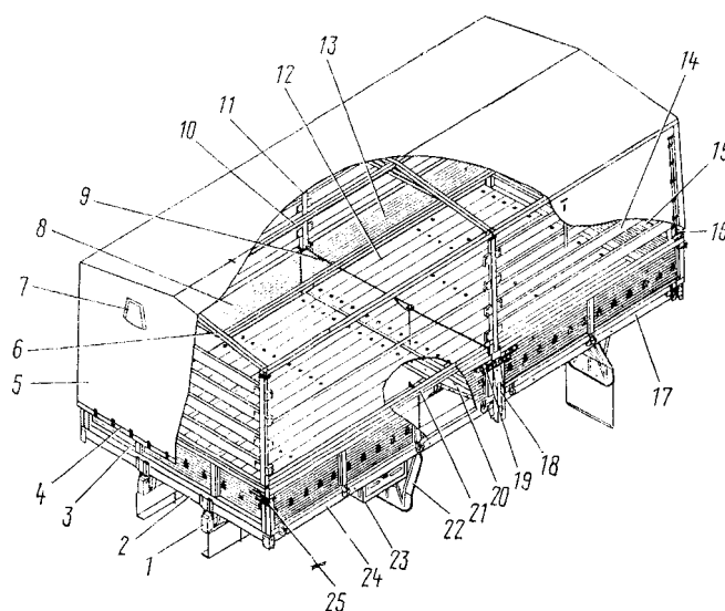
Рис. 259. Платформа автомобиля-тягача мод. 5320: 1 - брус основания продольный; 2 - балка передняя основания; 3 - борт передний; 4 - трос пломбирования; 5 - тент платформы; 6 - дуга каркаса тента; 7 - козырек вентиляционного люка; 8 - борт передний боковой; 9 - цепь стяжная стоек бортов; 10 - распорка стоек каркаса тента; 11 - стойка каркаса тента; 12 - щит настила пола; 13 - борт задний боковой; 14 - доска каркаса тента; 15 - борт задний; 16 - запор задней стойки каркаса тента; 17 - обвязка задняя боковая основания; 18 - стойка боковых бортов; 19 - запор боковой; 20 - балка поперечная каркаса основания; 21 - усилитель основания; 22 - брызговик; 23 - ящик инструментальный; 24 - обвязка передняя боковая; 25 - запор угловой бортов
