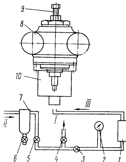
Рис. 101. Схема установки для испытаний пары шток-втулка: 1 - аккумулятор воздушный; 2 - манометр; 3, 4, 5, 6 - краны; 7 - масловлагоотделитель; 8 - корпус насоса; 9 - ограничитель перемещения штока; 10 - соединитель для подвода воздуха к корпусу насоса; I - в атмосферу; II - из системы; III - к насосу
