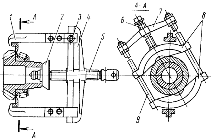
Рис. 189. Снятие внутреннего кольца подшипника ведущей конической шестерни заднего и промежуточного мостов, внутреннего кольца ведущей и ведомой конических шестерен: 1 - захват; 2 - наконечник; 3, 5, 6 - винты; 4, 7 - траверсы; 8 - клин; 9 - стойка
