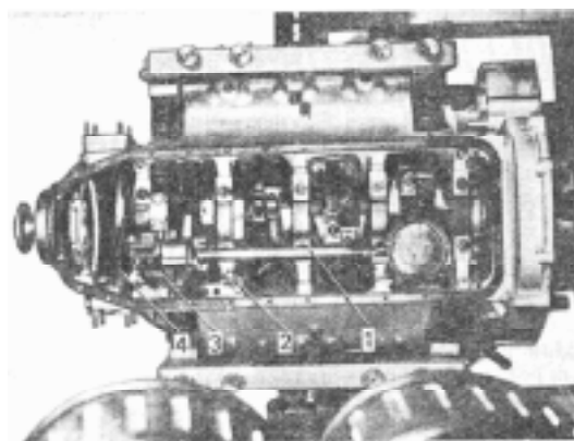
Рис. 98. Вид двигателя снизу со снятым масляным картером: 1 - трубка всасывающая; 2 - трубка подводящая клапана системы смазывания; 3 - насос масляный; 4 - шестерня ведомая привода масляного насоса
