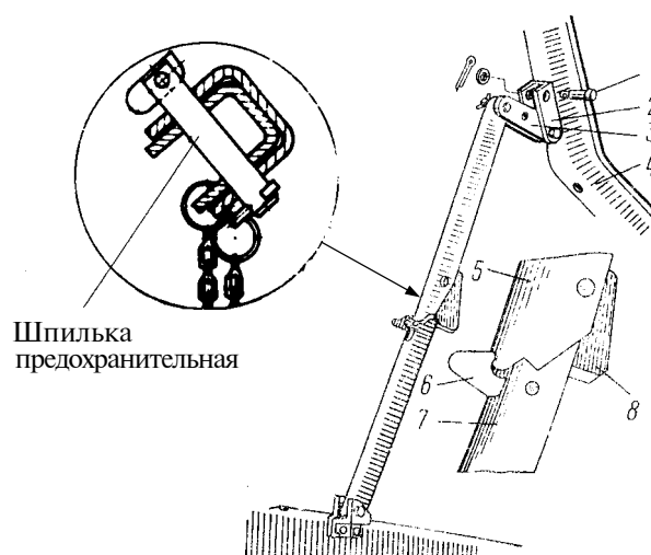
Рис. 246. Ограничитель подъема кабины: 1 - палец удлинителя; 2 - скоба верхняя; 3 - удлинитель; 4 - балка продольная пола кабины; 5 - стойка верхняя; 6 - крючок-зашелка; 7 - стойка нижняя; 8 - буфер
