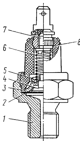
Рис. 313. Датчик падения давления: 1 - корпус; 2 - мембрана; 3 - контакт неподвижный; 4 - толкатель; 5 - контакт подвижный; 6 - пружина; 7 - винт регулировочный; 8 - изолятор
