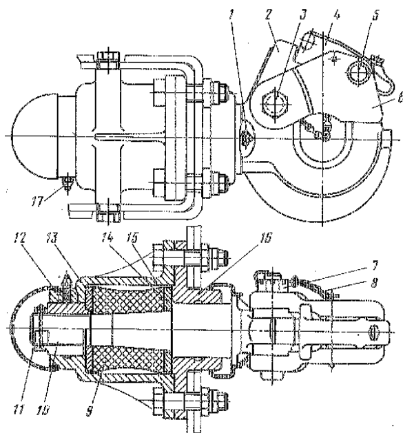
Рис. 199. Тягово-сцепное устройство: 1, 17 — масленки; 2 — крюк с грязеотражателем; 3 — ось защелки крюка; 4 — собачка защелки; 5 — ось собачки; 6 — защелка; 7 — гайка; 8 — цепь шплинта замка; 9 — упругий элемент; 10 — гайка крюка; 11 — шплинт; 12 — защитный колпак; 13, 14 — фланцы; 15 — корпус; 16 — крышка корпуса
