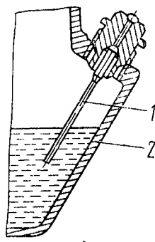
Рис. 142. Положение указателя уровня масла при замере: 1 - указатель уровня масла с пробкой; 2 - картер коробки передач
