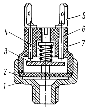
Рис. 314. Датчик включения сигнала торможения: 1 - корпус; 2-мембрана; 3 - контакт неподвижный; 4 - пружина; 5 - вывод неподвижного контакта; 6 - контакт неподвижный; 7 - крышка
