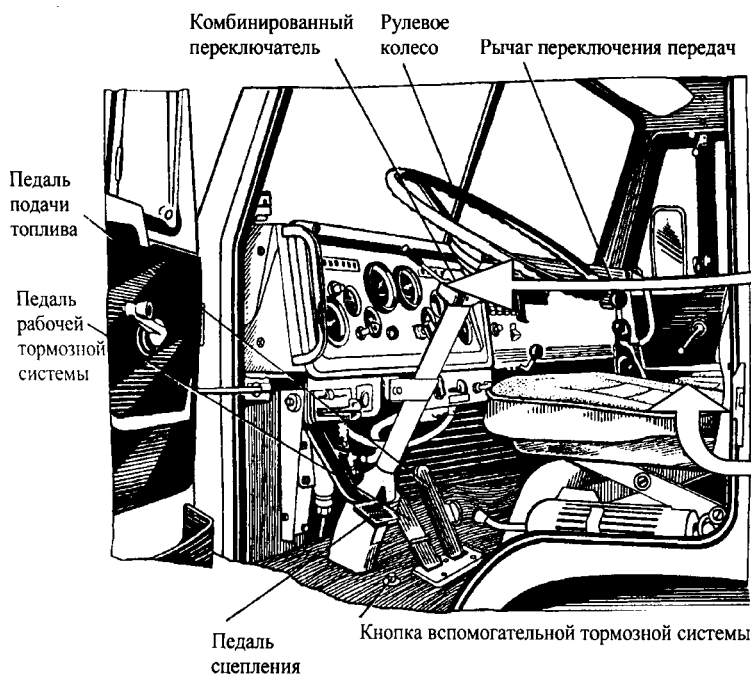
Рис. 1. Кабина
