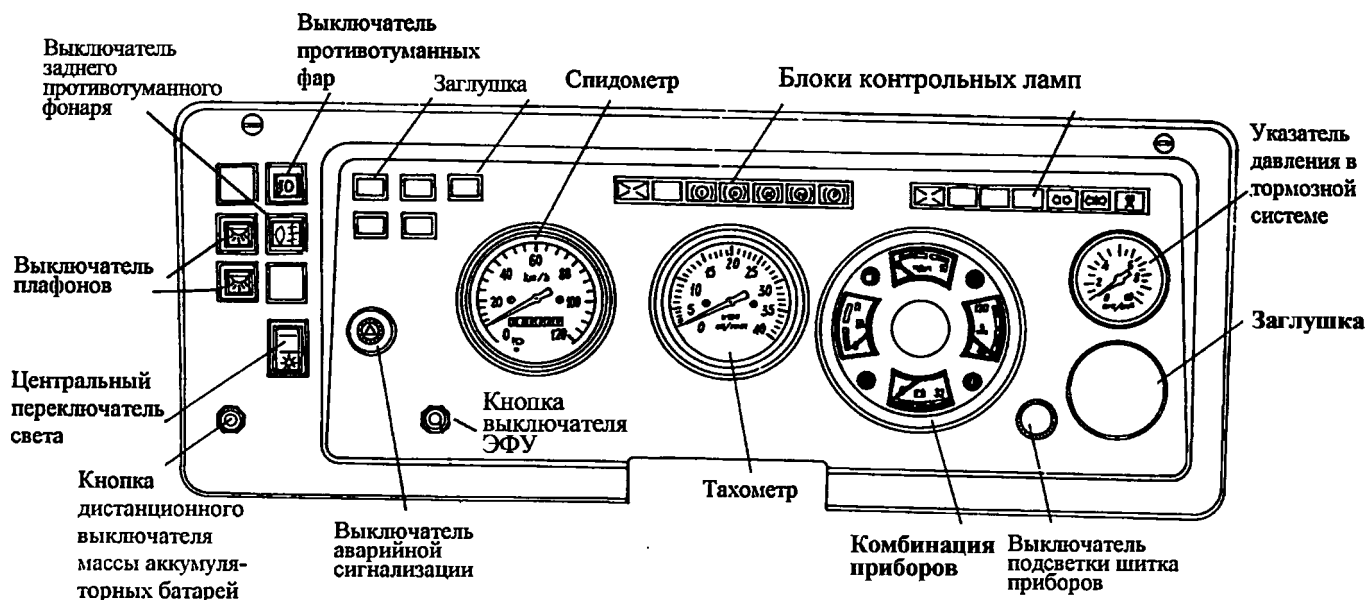
Рис. 5. Щиток приборов
