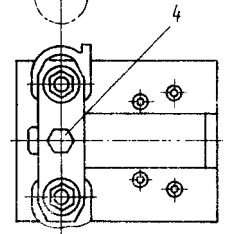
Рис. 105. Разборка форсунки в приспособлении И801.20.000: 1 - упор; 2 - станина; 3 - форсунка; 4 - болт
