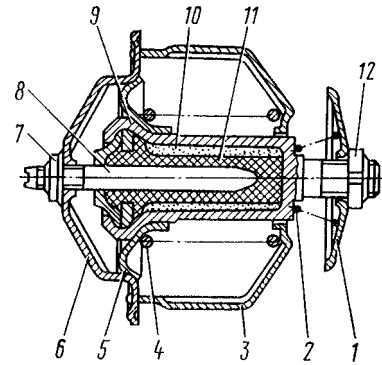
Рис. 57. Термостат: 1, 5 - клапаны; 2, 4 - пружины; 3, 6 - стойки; 7, 12 - гайки регулировочные; 8 - шток; 9 - баллон; 10 - масса активная (церезин); 11 - вставка резиновая с шайбой
