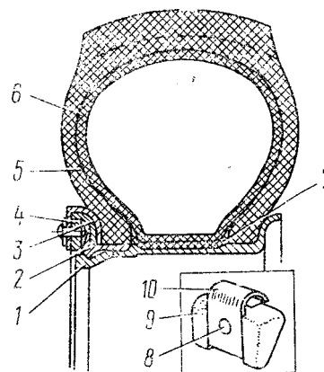
Рис. 214. Колесо с балансировочными грузами: 1 - обод колеса; 2 - кольцо замочное; 3 - кольцо бортовое; 4 - груз балансировочный в сборе; 5 - шина; 6 - камера; 7 - лента ободная; 8 - заклепка; 9 - груз балансировочный; 10 - пружина
