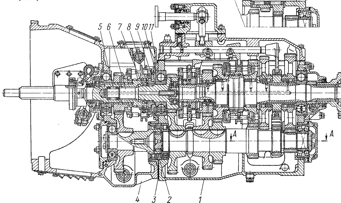
Рис. 136. Коробка передач десятиступенчатая модели 15: 1 - коробка передач основная пятиступенчатая; 2 - втулка распорная; 3 - прокладка уплотнительная; 4 - делитель передач; 5 - подшипник передний роликовый ведущего вала; 6 - вал ведущий; 7 - гайка кольцевая; 8 - шайба; 9 - муфта синхронизатора; 10 - прокладки регулировочные; 11 - крышка заднего подшипника ведущего вала
